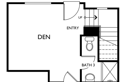
OPTION Optional Den at Bedroom 3
